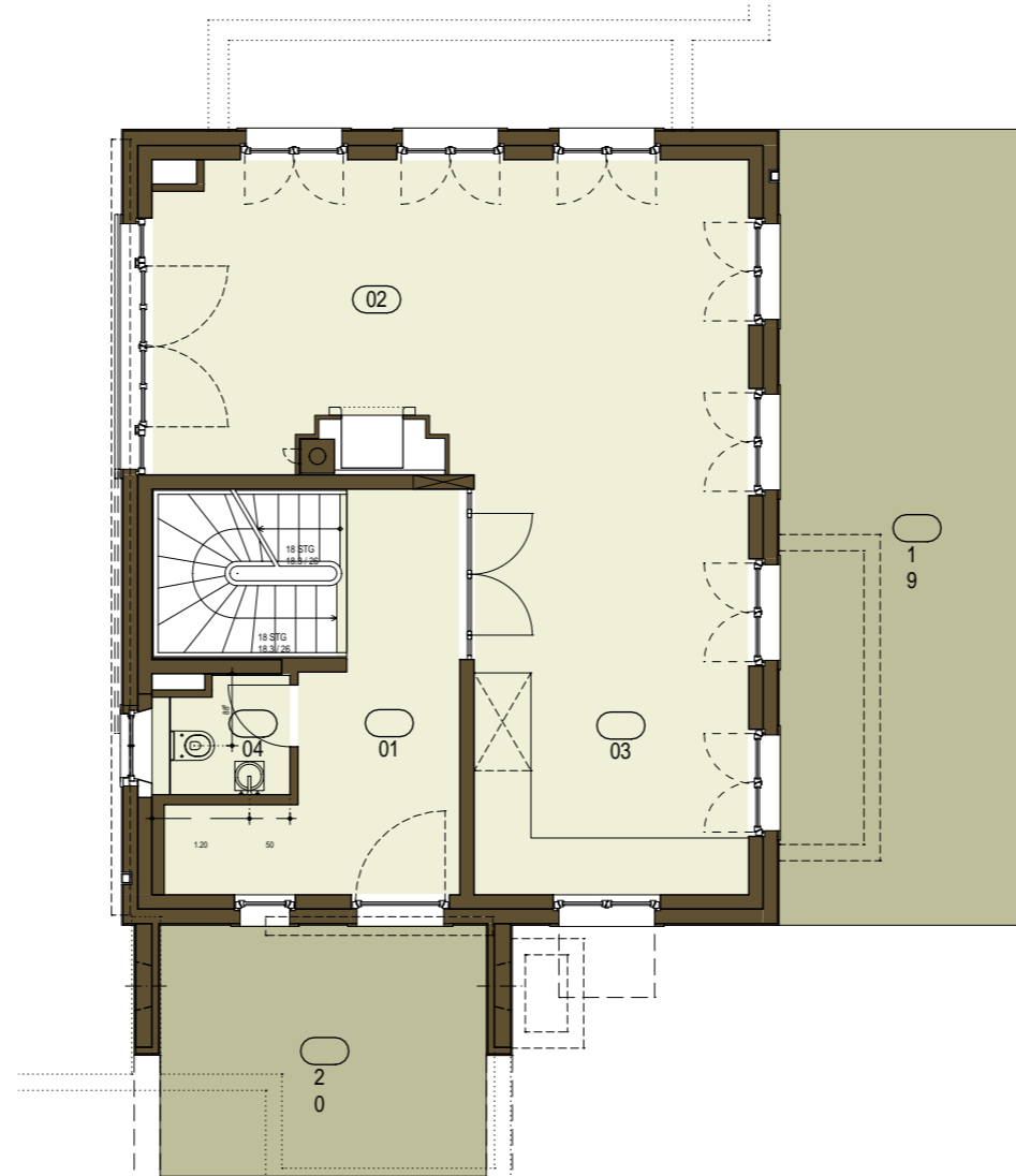
ERDGESCHOSS
