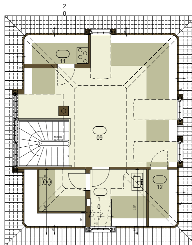
DACHGESCHOSS
