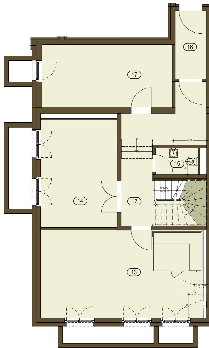
UNTERGESCHOSS
