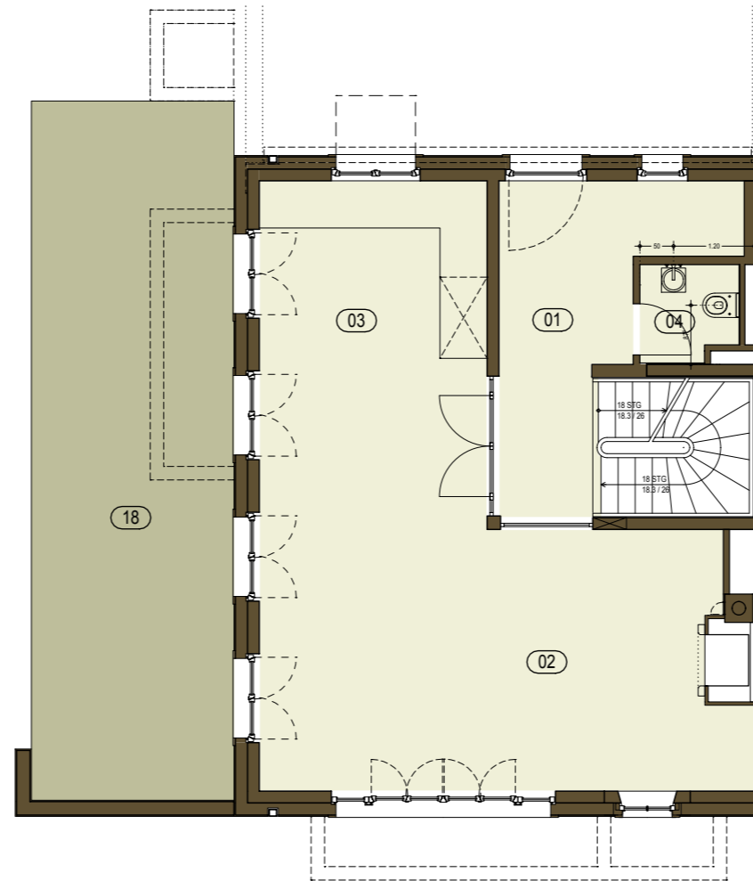
ERDGESCHOSS
