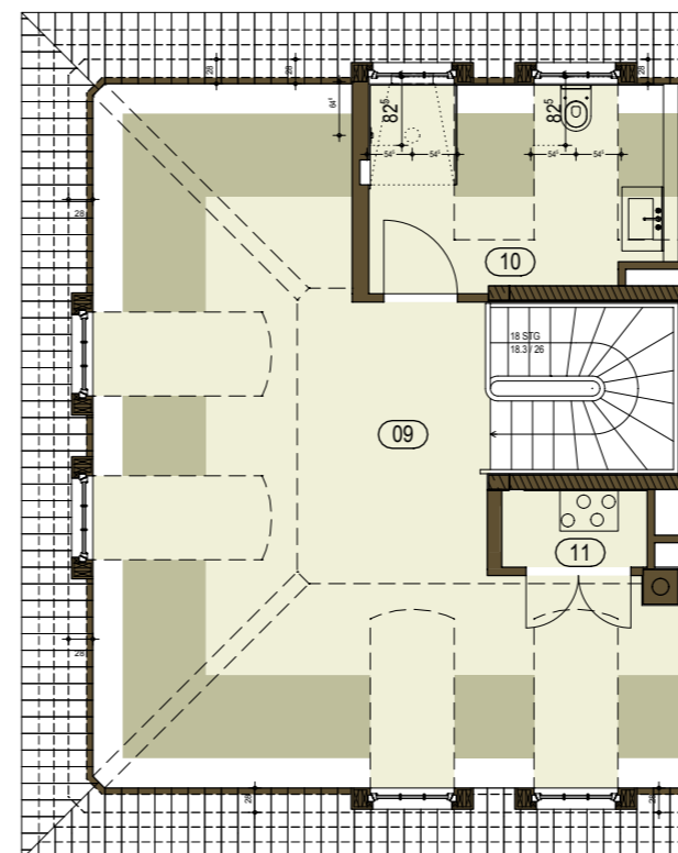
DACHGESCHOSS
