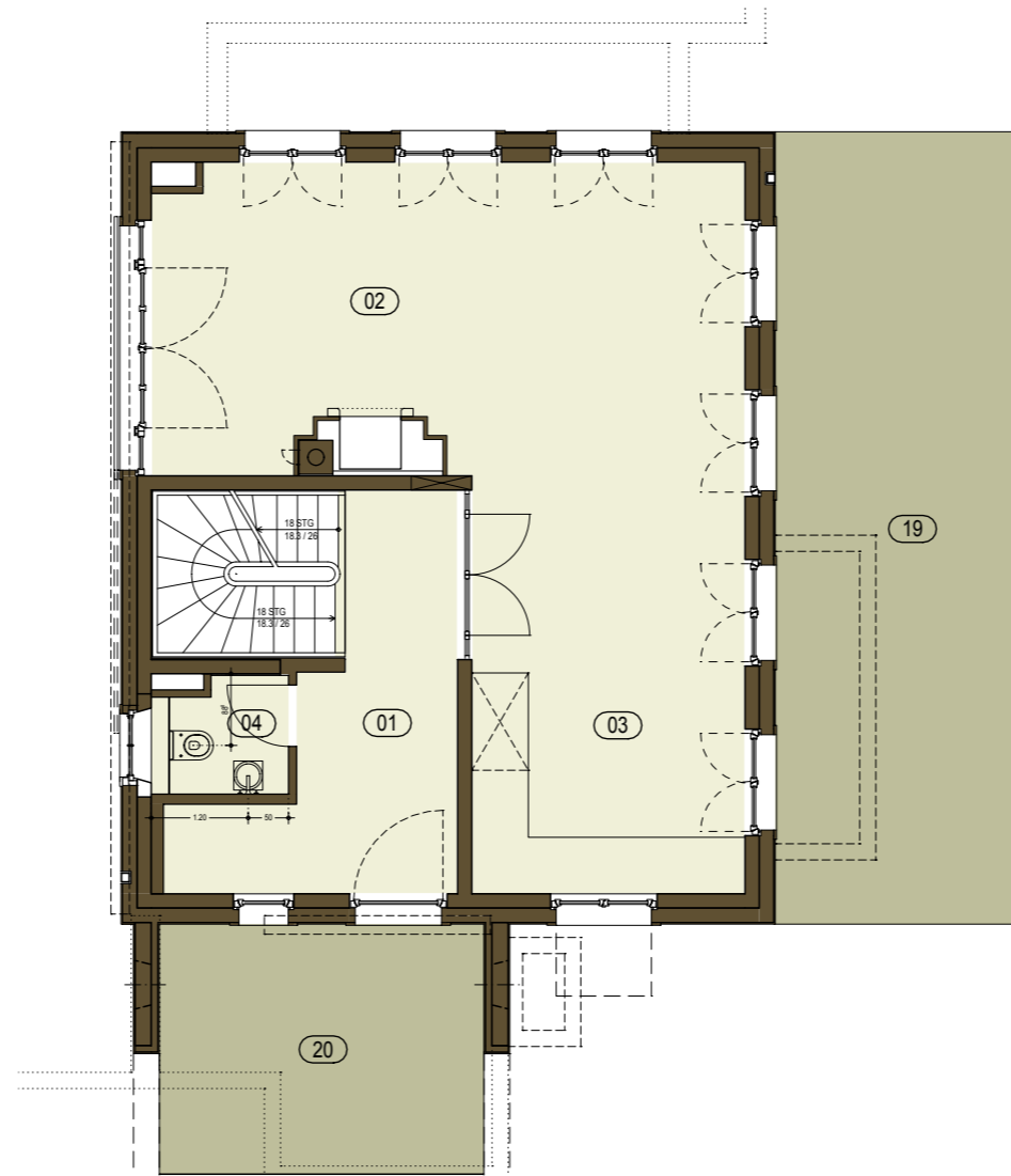
ERDGESCHOSS
