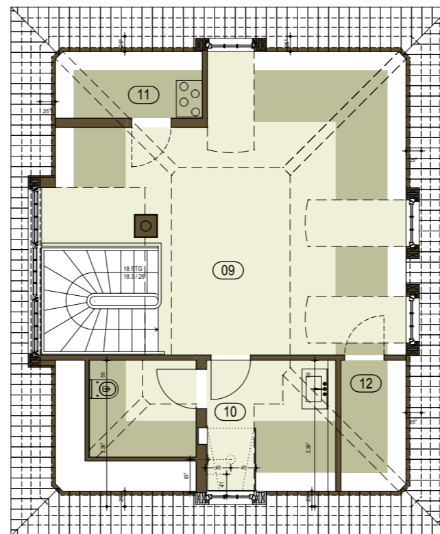
DACHGESCHOSS
